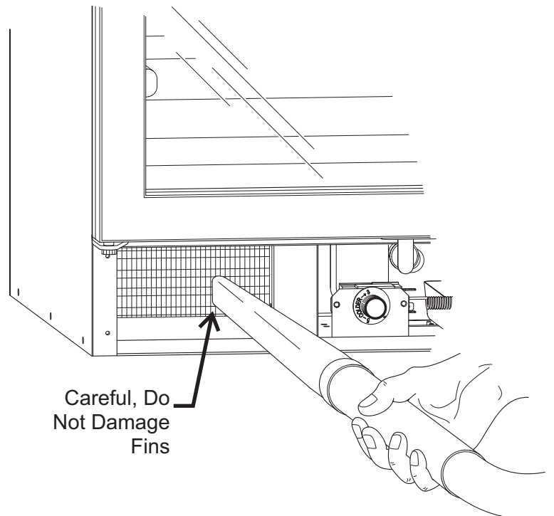
Vacuum Fins
