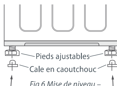
Fig.6 Mise de niveau – Étapes 1 et 2
