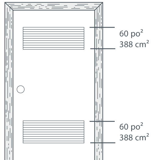
Fig.11 Porte-persienne pour laveuse et sécheuse
