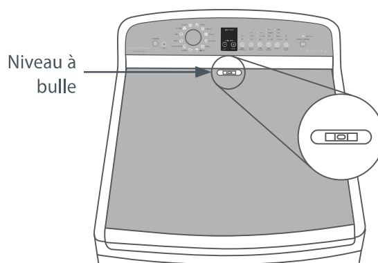
Fig.7 Mise de niveau – Étape 4
