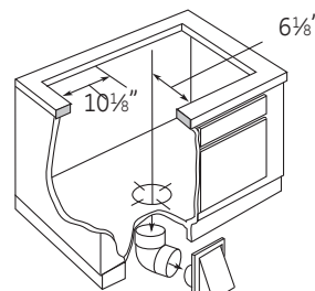
Ventilación vertical
