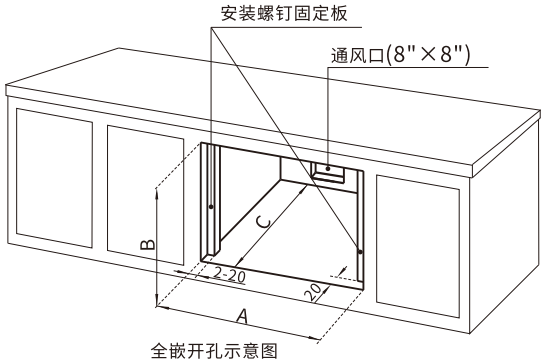
全嵌开孔示意图
