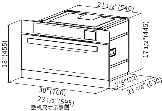
整机尺寸示意图
