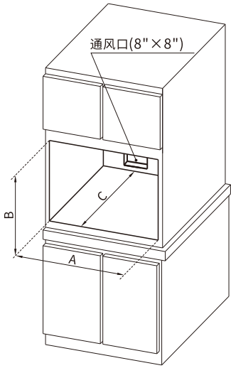
半嵌开孔示意图
