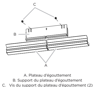
C. Vis du support du plateau d'égouttement (2)
