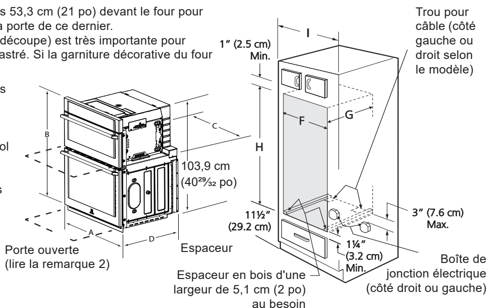
Figure 1: Dimensions du produit et de l'ouverture
