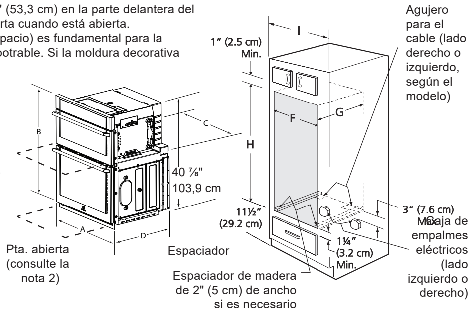
Figure 1: Dimensiones del producto y del corte
