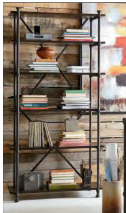
Left: 400-101 Home Office Steel Bookcase-KD W34 D18 H76 Six fixed shelves (from top to bottom): W34 D18 H10½ W34 D18 H12 W34 D18 H14 W34 D18 H14 W34 D18 H15½
