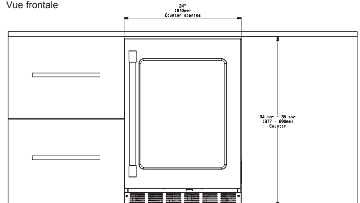
Vue frontale
