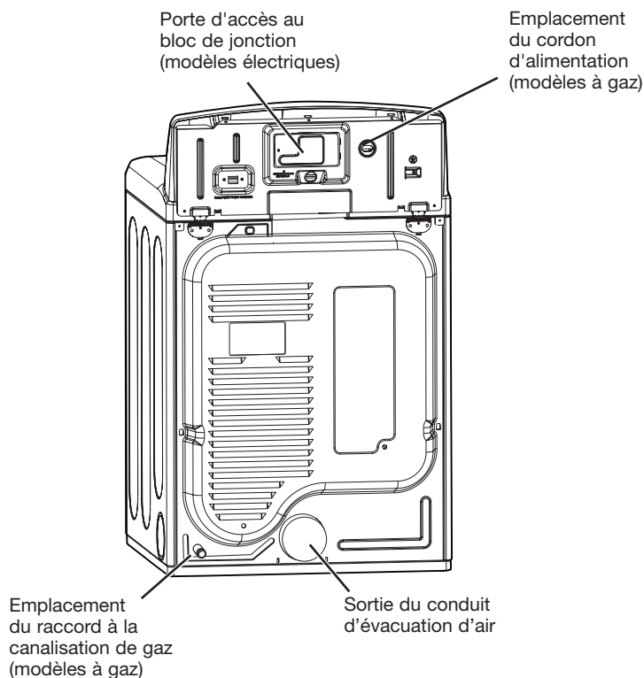
Dos de la sècheuse
