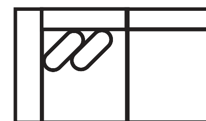
2487-0723 LHF Loveseat L-75" x D-39" x H-34"
