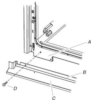
A. Oven frame B. Vent tab C. Bottom vent D. #8-18 x \frac{3}{8} screws
