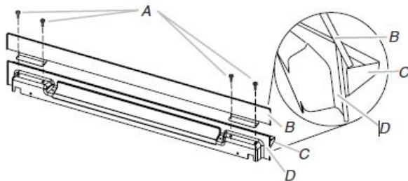
A. Vis n° 8-18 x \frac{1}{4} po (6,4 mm) B. Garniture de l'évent inférieur C. Pièce d'évent supérieure D. Pièce d'évent inférieure
