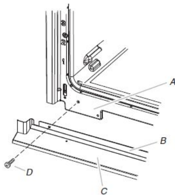
A. Marco del horno B. Lengüeta de ducto de ventilación C. Ducto de ventilación del horno D. Tornillos n.º 8-18 x \frac{3}{8} " (9,5 mm)
