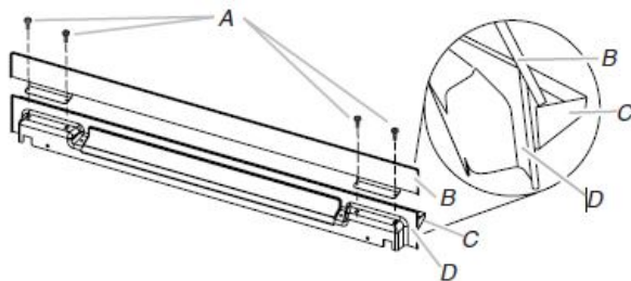
A. Tornillos n.º 8-18 x \frac{1}{4} " (6,4 mm) B. Borde de ducto de ventilación inferior C. Pieza superior del ducto de ventilación D. Pieza inferior del ducto de ventilación
