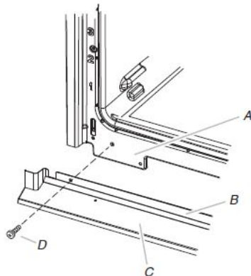
A. Châssis du four B. Support de l'évent C. Évent du four D. Vis n° 8-18 x \frac{3}{8} po (9,5 mm)
