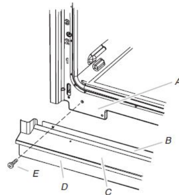
A. Marco del horno B. Lengüeta de ducto de ventilación C. Ducto de ventilación del horno D. Borde de ducto de ventilación inferior E. Tornillo n.º 8-18 x \frac{3}{8} " (9,5 mm)
