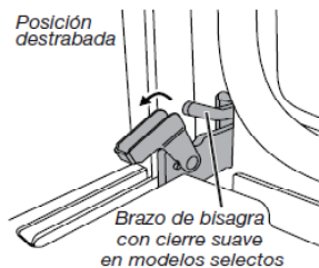
A. Traba de bisagra de la puerta del horno en posición parcialmente destrabada
