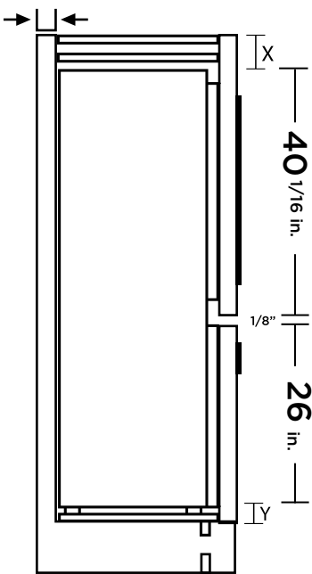
DOOR PANEL DIMENSIONS
