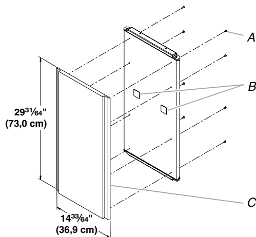
A. Vis à bois n° 8 x \frac{1}{2} ", tête bombée B. Patins adhésifs C. Panneau personnalisé
