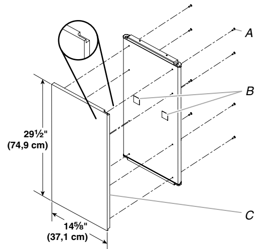
A. Vis à bois n° 8 x \frac{1}{2} ", tête bombée B. Patins adhésifs C. Panneau personnalisé
