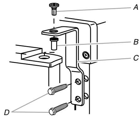
A. Pasador de la bisagra B. Funda del pasador de la bisagra C. Bisagra D. Tornillo de cabeza hexagonal para bisagra
