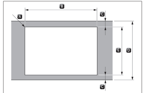
Fig. 11.6 Dimensions de découpe pour montage en saillie
