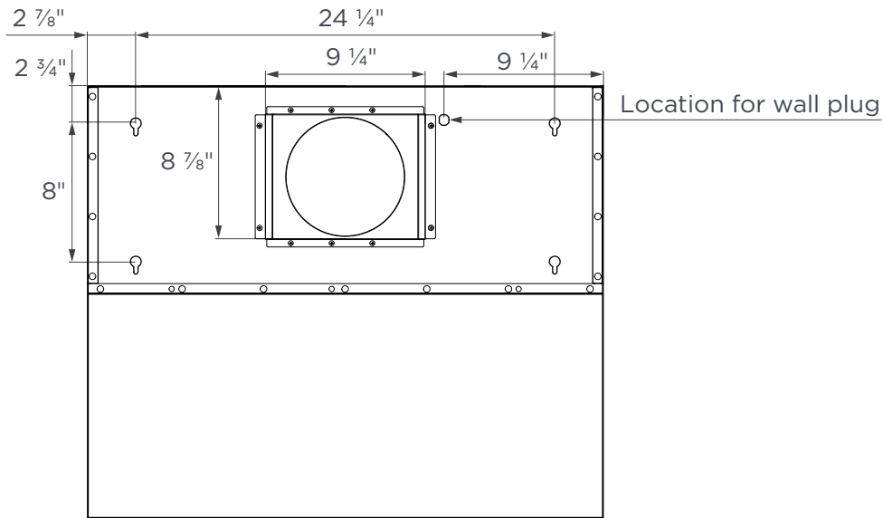
TOP
