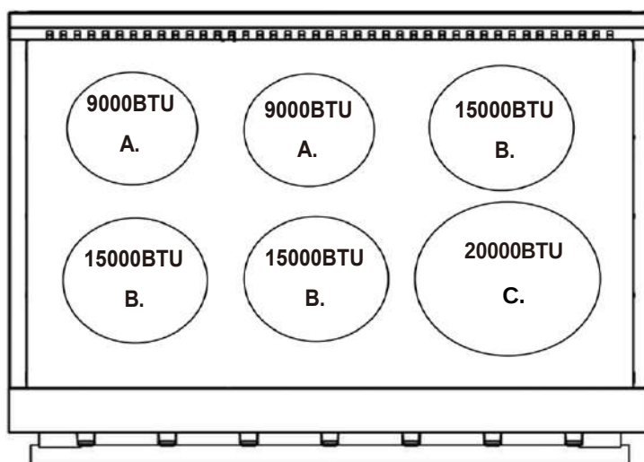
Modèle: FFSGS6156-36 FFSGS6156-36BLK FFSGS6156-36WHT
