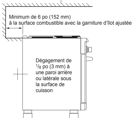
Dégagements pour l'installation en présence d'un dossieret
