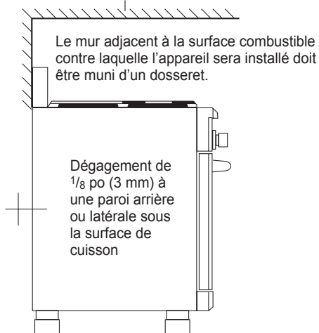
Dégagements pour l'installation en présence d'une garniture d'évent
