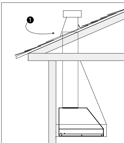
① Pente du toit avec solin et capuchon
