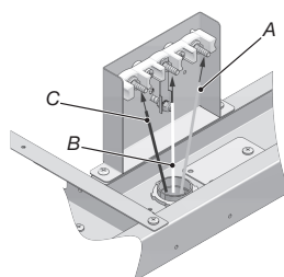
(tipo A horizontales) CONEXIÓN 3 HILOS
