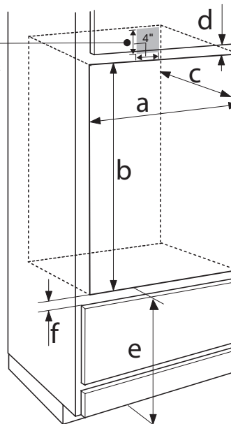
Four double : installé dans un placard
