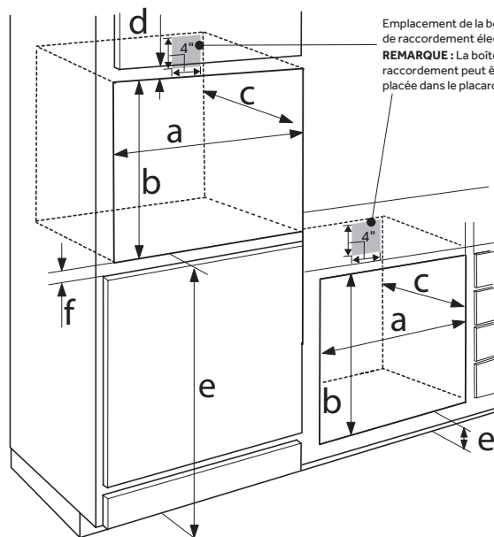
Four simple : installé dans un placard et sous le comptoir
