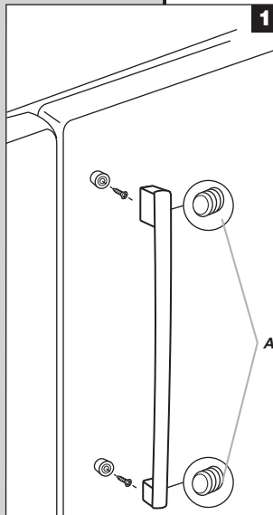
A. Vis de retenue de \frac{3}{32} " ou \frac{1}{8} "
