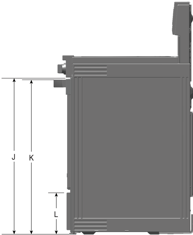
VUE LATÉRALE
