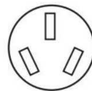
Tomacorriente de 3 hilos (10-50R)
