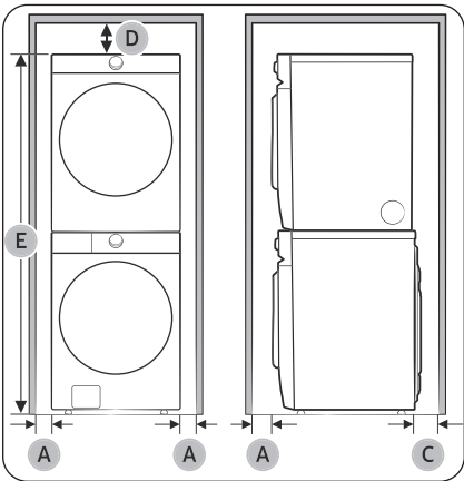
Installation superposée (Modèle : SKK-9MC*)
