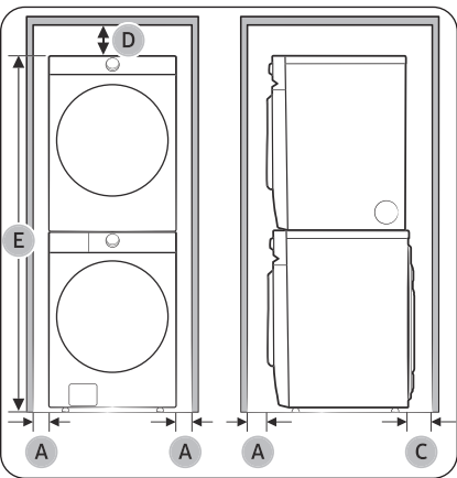
Instalación apilada (Modelo: SKK-9MC*)
