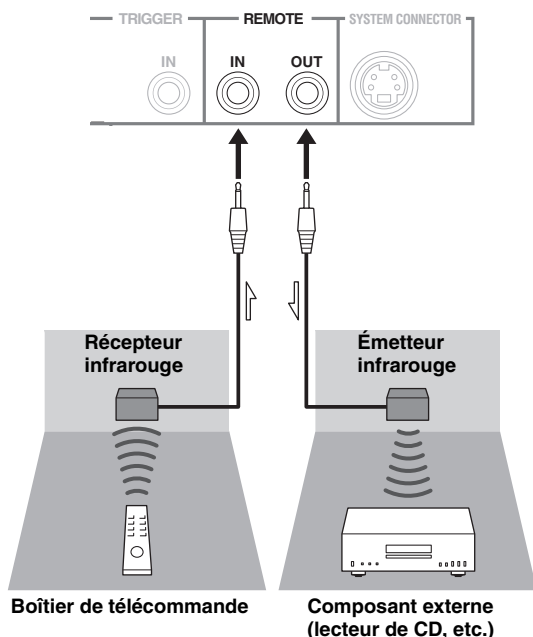
Panneau arrière de l'A-S2100
