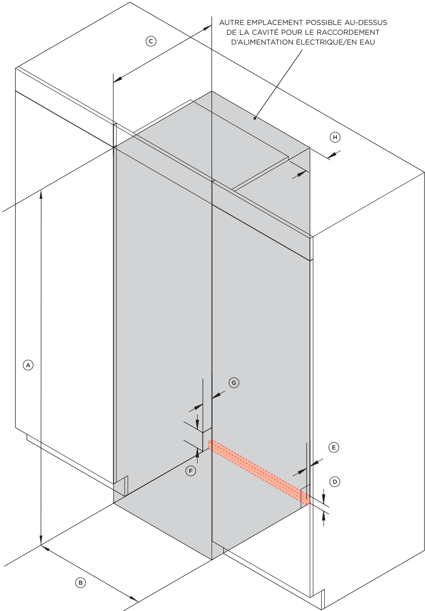
VUE DE BIAIS
