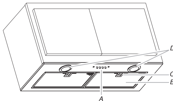
A. Commandes du ventilateur et de lampes DEL B. Filtre à graisse C. Poignée du filtre à graisse D. Logements des lampes DEL
