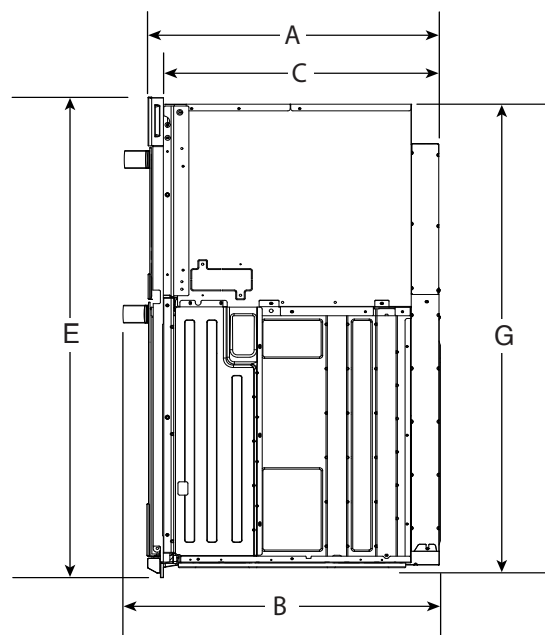
VISTA LATERAL
