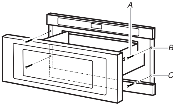
A. (4) Vis de montage de 1 po (2,5 cm) B. Trous de vis du rebord de montage C. Rebord de montage
