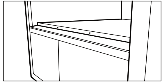
Détail de la tablette montrant le déflecteur d'évacuation installé.
