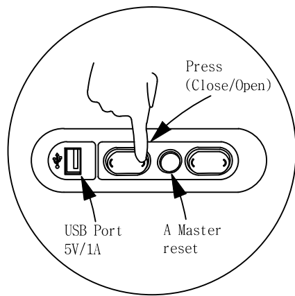
Headrest
