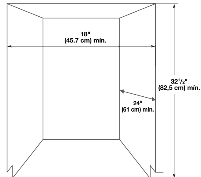
Dimensiones de corte
