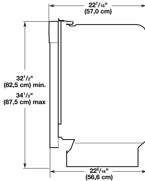
Vue latérale du panneau de porte en métal de 18"
