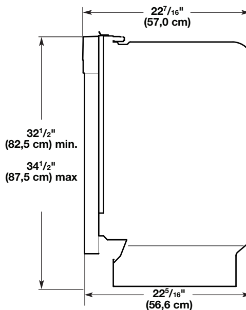
Vue latérale du panneau de porte en métal de 24"
