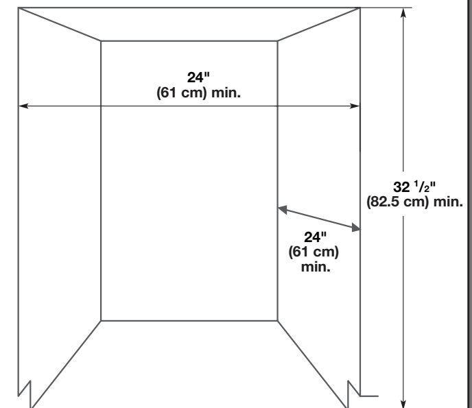
Cutout Dimensions
