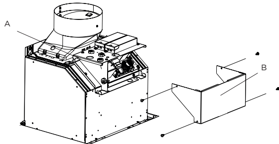
A. Opercule arrachable B. Couvercle du boîtier
