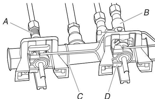
A. Valve en aluminium pour les brûleurs arrière gauche, arrière droit, arrière central et avant central
