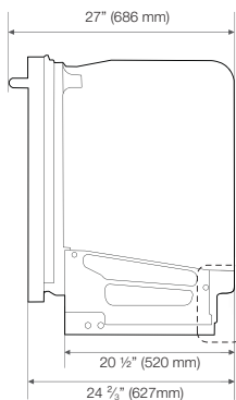
Vista lateral (Serie DMT800 / Serie DMT610 / Serie DMT400)
