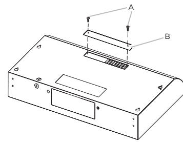
A. Tornillos (2) B. Cubierta de la salida recirculante
