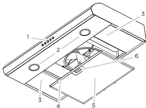
1. Controles 2. Lámparas LED 3. Paneles laterales 4. Estafa del filtro de grasa 5. Filtro de grasa 6. Manija del filtro de grasa
