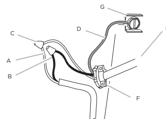
A. Alambres blancos B. Alambres negros C. Conectores de alambres aprobados por UL D. Alambres verdes (o desnudos) - verdes de puesta a tierra E. Cable de alimentación o kit de accesorios del cable de alimentación F. UL listed or CSA approved 1/2" strain relief G. Tornillo de tierra verde
