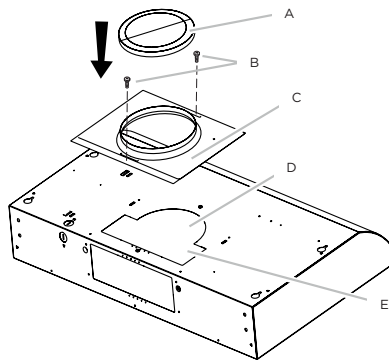
A. Válvula redonda de 7" (17.8 cm) B. Tornillos metálicos C. Transición redonda de 7" (17.8 cm) D. Precorte de ventilación redonda E. Precorte de ventilación rectangular
