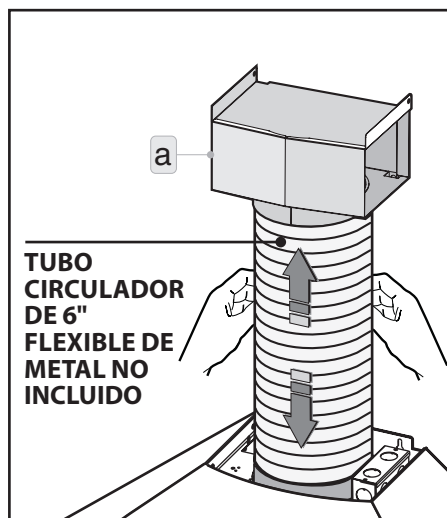
Fig.4: Una vez que se introduzca el deflector en la brida y se fije a la pared, conecte el tubo flexible ( TUBO CIRCULADOR DE 6" FLEXIBLE DE METAL NO INCLUIDO ) al deflector, utilice una cinta para sellar.
