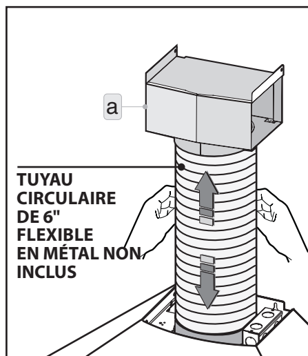
Fig.4: Après avoir introduit le déflecteur dans l'étrier et l'avoir fixé au mur, raccorder le tuyau flexible ( TUYAU CIRCULAIRE DE 6\"
