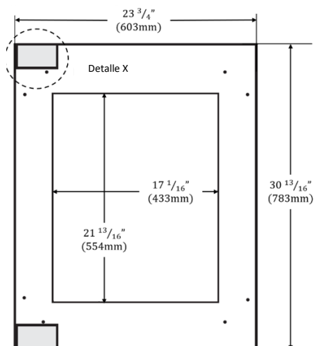
Placa base - Vista posterior
