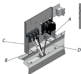
(tipo B) CONEXIÓN 4 HILOS
