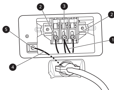
① Fil blanc déplacé de la vis de masse
