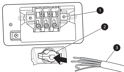
① Bloc du terminal
