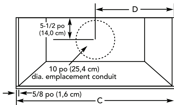
Installation de ventilateur en ligne ou 900 ou 1200 CFM extérieur Modèles de 36 po, 42 po de largeur
