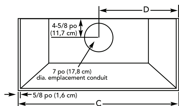
Installation de ventilateur 300 ou 600 CFM intérieur Modèles de 36 po, 42 po de largeur
