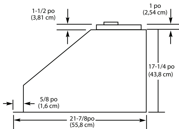
Pour installation de 900, 1200 ou 1500 CFM extérieur ou installation de ventilateur en ligne
