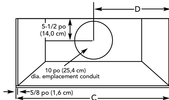
Installation de ventilateur intérieur 1200 CFM Modèles de 36 po, 42 po, 48 po, 60 po de largeur
