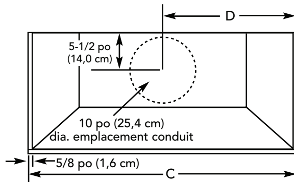
Installation de ventilateur en ligne ou extérieur 1200 ou 1500 CFM Modèles de 48 po, 60 po de largeur
