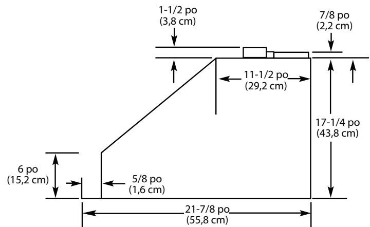
Pour installation de ventilateur 300, 600 ou 1200 CFM intérieur
