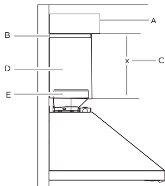
A. Déflecteur d'air B. Bride pour conduit C. X = longueur à laquelle couper le conduit d'évacuation D. Conduit d'évacuation E. Sortie d'évacuation
