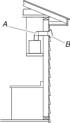
Évacuation par le mur
