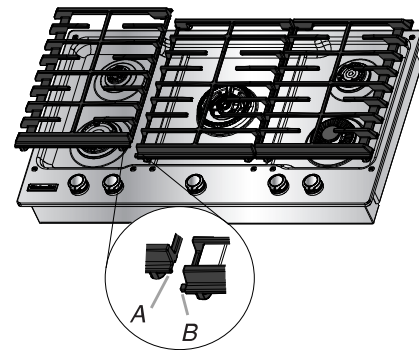
A. Encoche de la grille externe B. Onglet de la grille centrale
