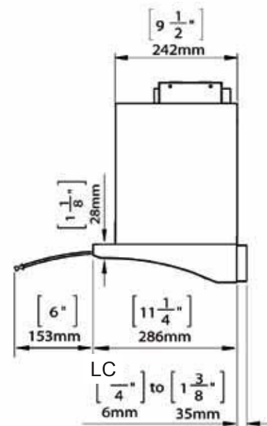
Côté de la hotte
