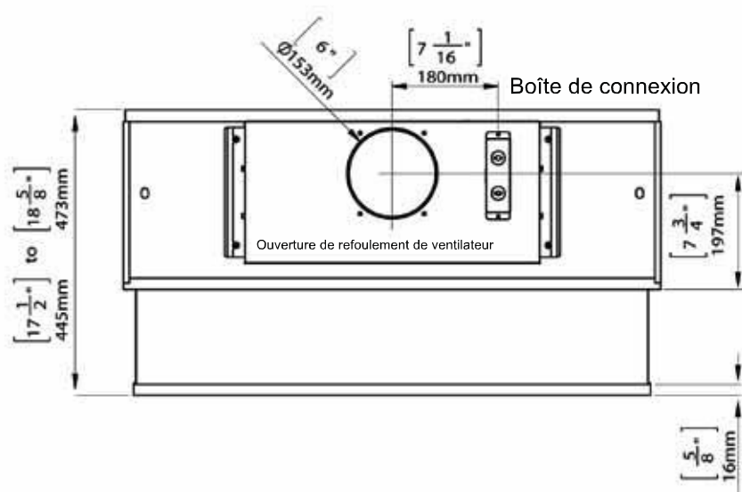
Dessus de la hotte
